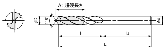
工具径φD Tool dia.φD 許容差 Tolerance 5.0以上6.0以下 5.0 Over 6.0 Up to 0 -0.018 6.0をこえ10.0以下 6.0 Over 10.0 Up to 0 -0.022 10.0をこえ18.0以下 10.0 Over 18.0 Up to 0 -0.027 18.0をこえ30.0以下 18.0 Over 30.0 Up to 0 -0.033 30.0をこえ40.0以下 30.0 Over 40.0 Up to 0 -0.039
