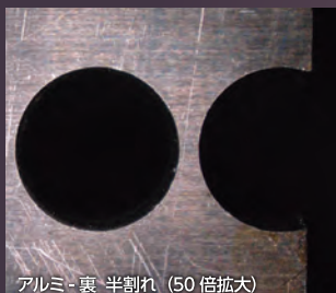
アルミ-裏 半割れ (50倍拡大)
