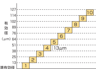
タフレットの精度番号の有効径位置
