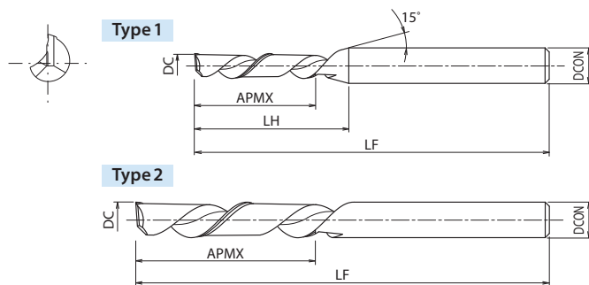
DLC-E1-5D-L 5D刃長 (右刃左ねじれ溝)
