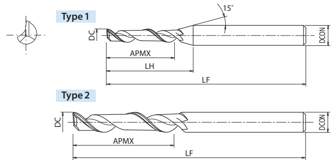
DLC-E1-5D 5D刃長
